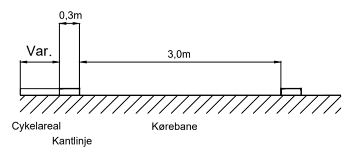
2 minus 1-vej, tværsnit
